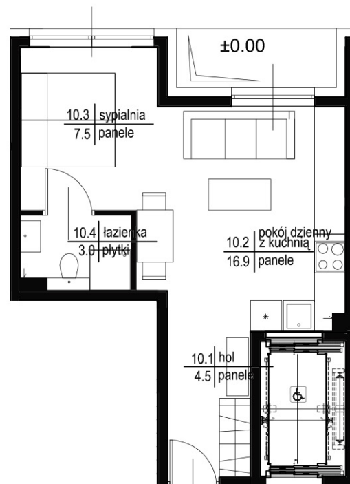
MIESZKANIE 10- 31.9 m 2
