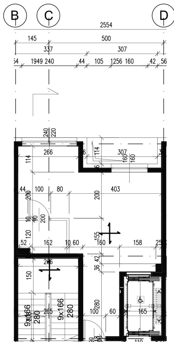
MIESZKANIE 10- 31.9 m 2
